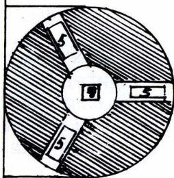
Vandret snit af Fyrkanaler.
