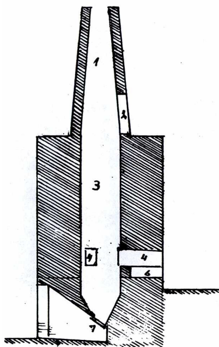
Lodret snit af Kalkovn.
